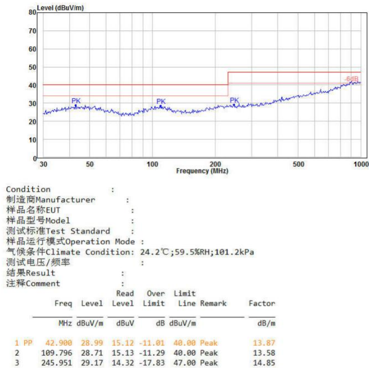
图 6-6 RE 测试垂直方向
