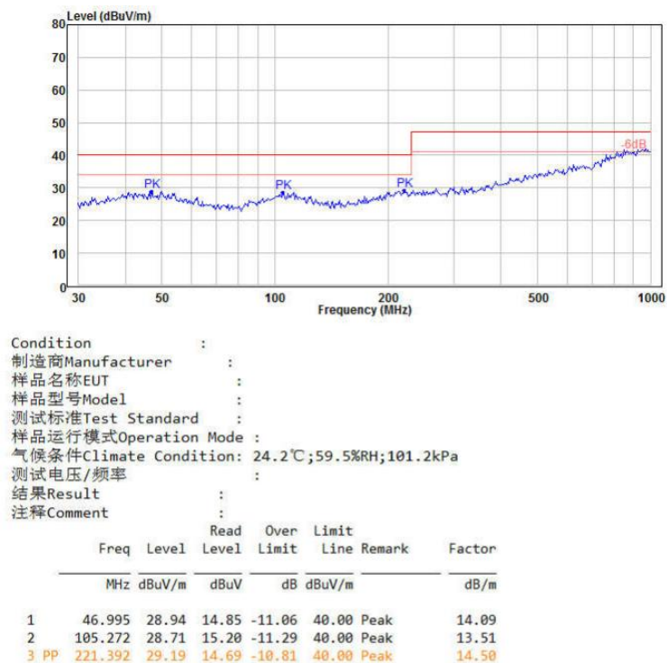
图 6-5 RE 测试水平方向
