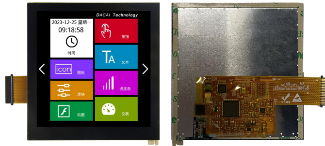
图 1-1 4.0 寸电容触摸参考图
