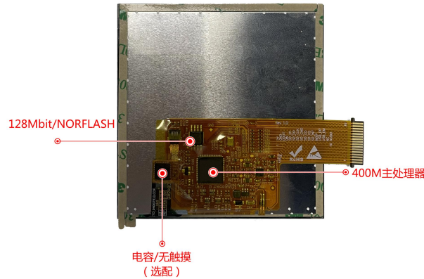
图 1-3 硬件配置图
